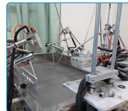
壽命 & 流水測試
